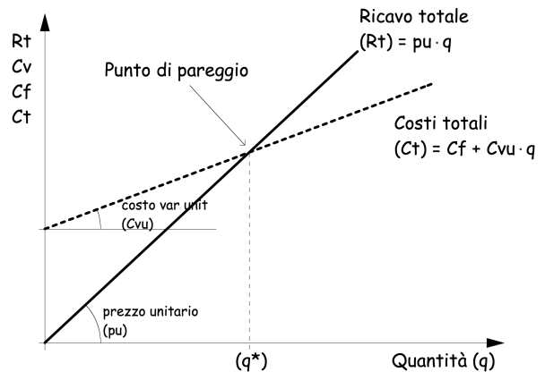
PROFITTO TOTALE e COSTI TOTALI CON ANDAMENTO SEMPLIFICATO LINEARE = PUNTO DI PAREGGIO
